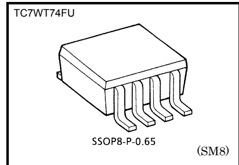
Weight SSOP8-P-0.65: 0.02 g (typ.)
